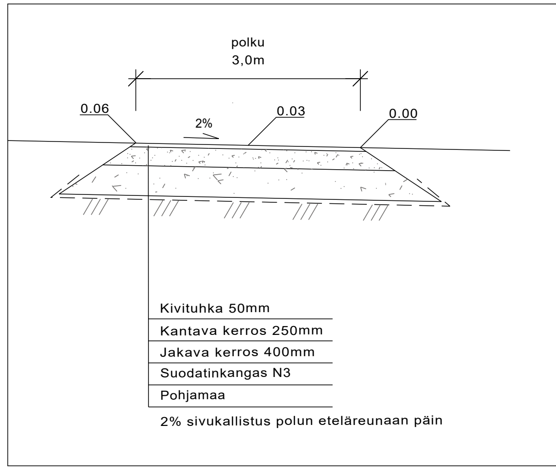
KIVITUHKAPOLUN TYYPPIPOIKKILEIKKAUS 1:50
