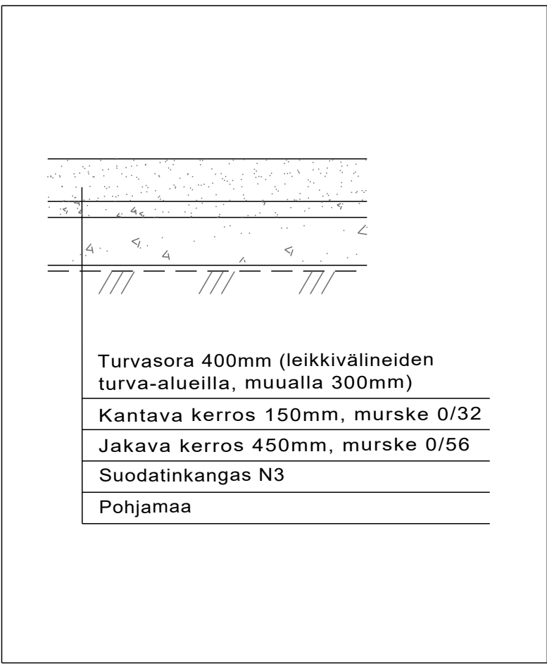
TURVASORA-ALUEEN TYYPPIPOIKKILEIKKAUS 1:50
